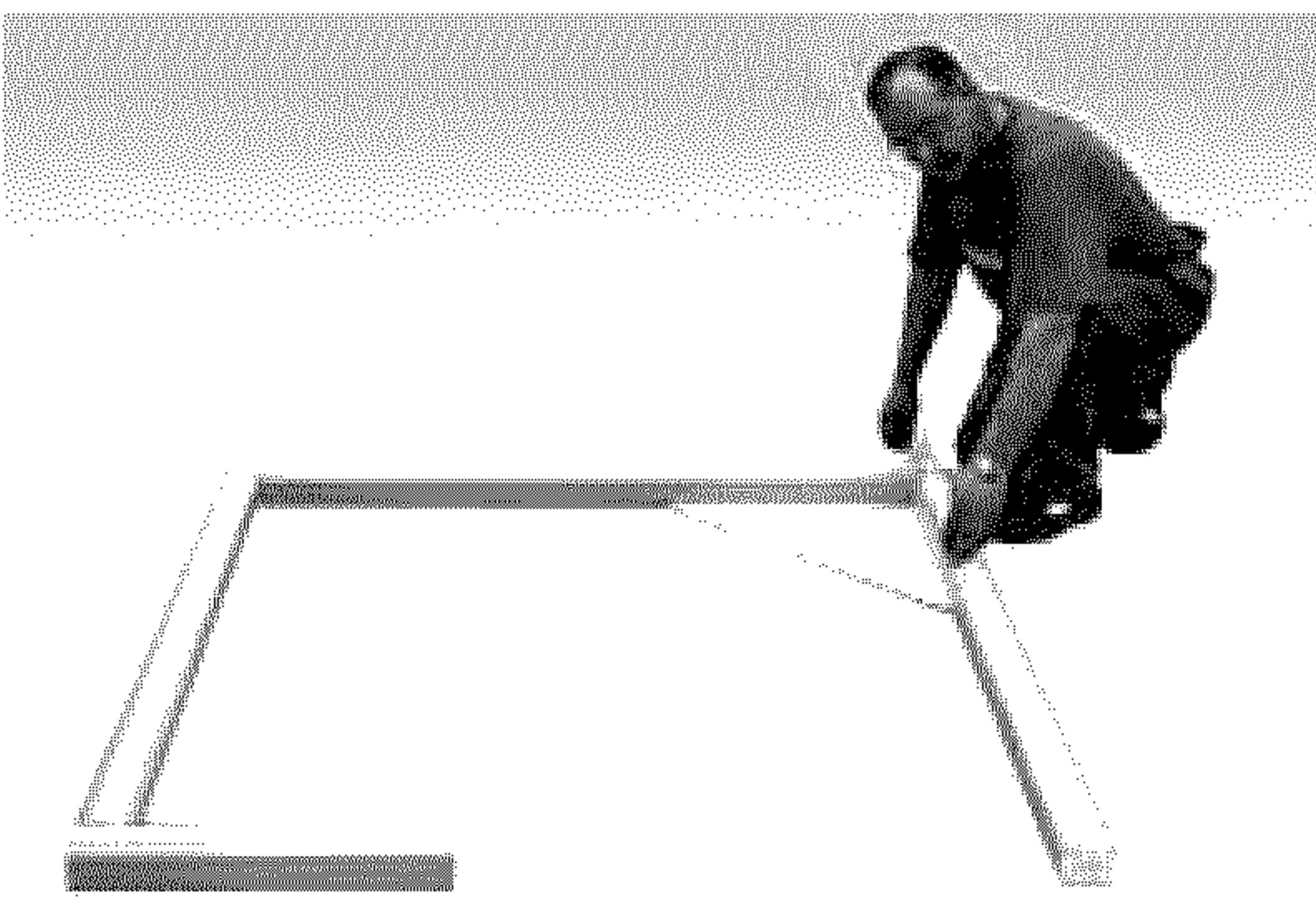
Рис.4 Монтаж цоколя, контроль углов.
