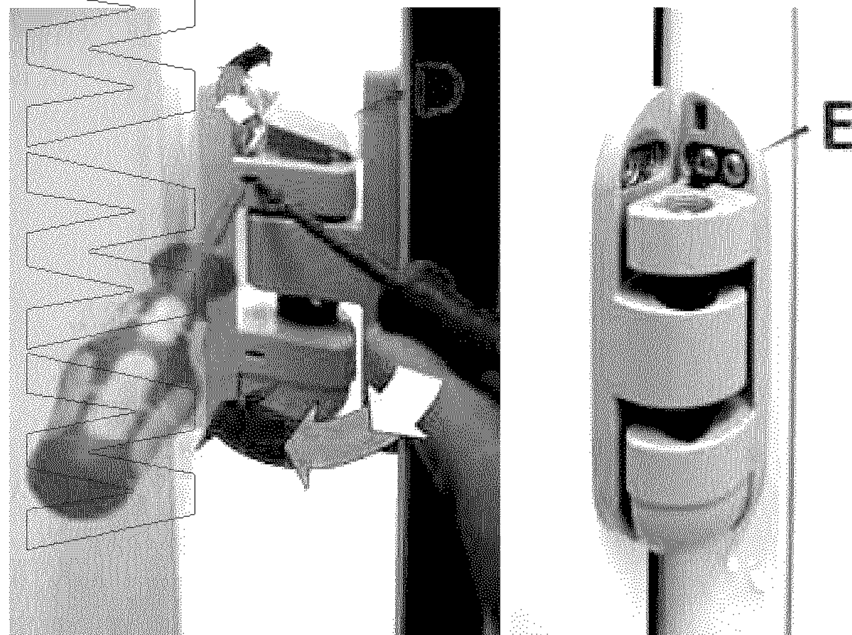
Рис.13 Монтаж петли.
