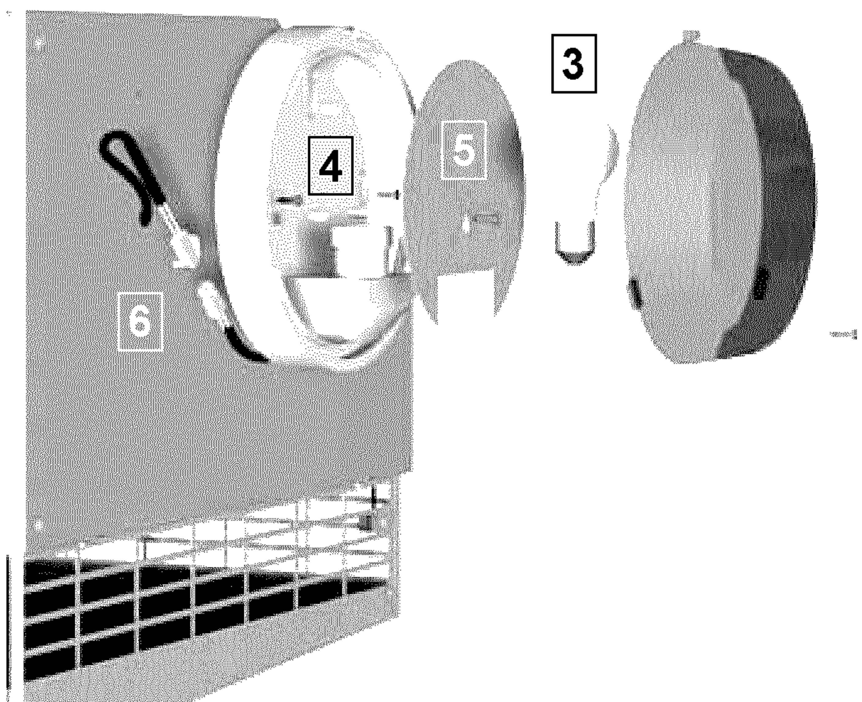
Рис.11b Установка светильника.
